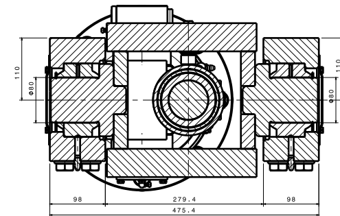
Vista in sezione D-D Scala: 4:9
