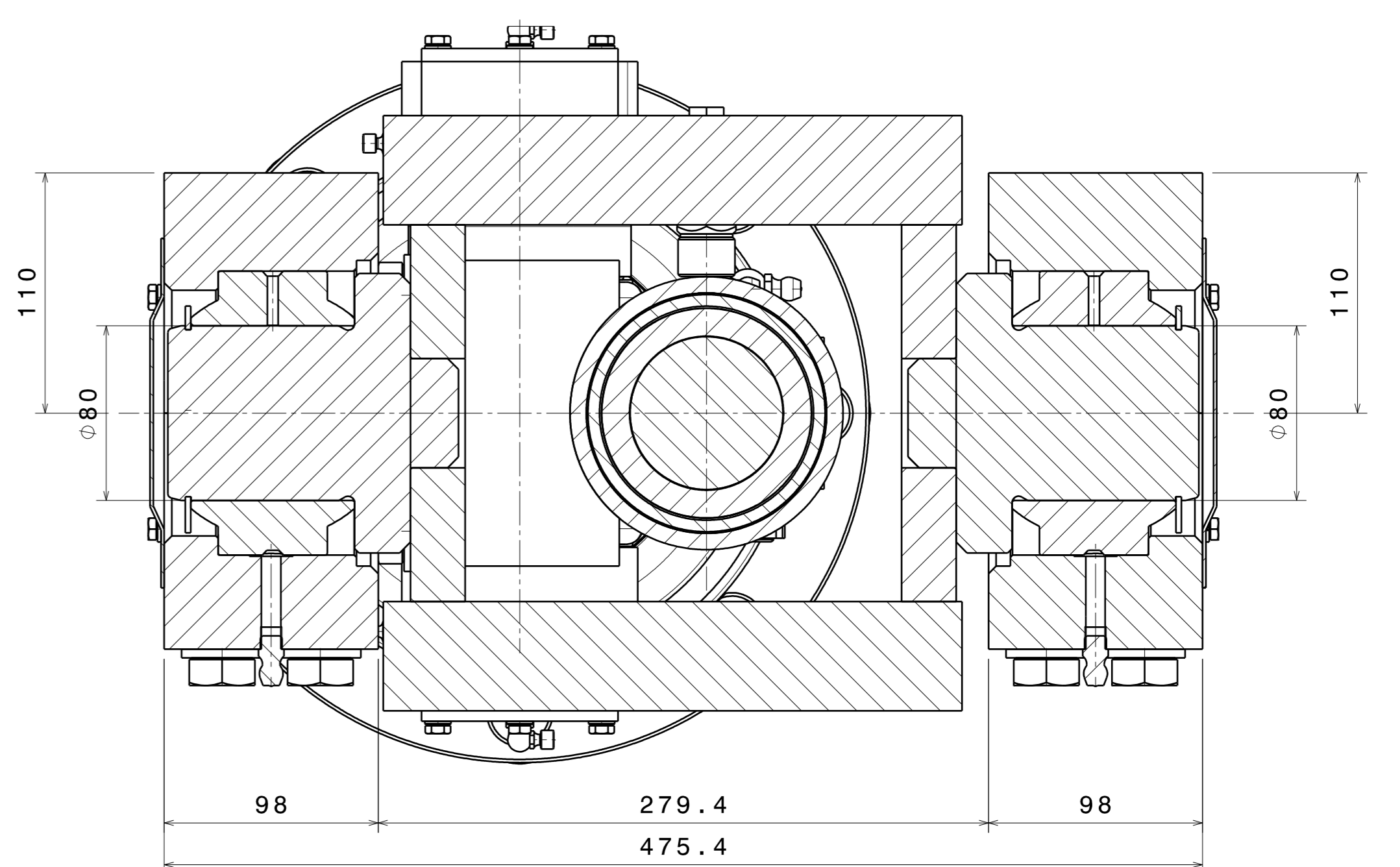
Vista in sezione D-D Scala: 4:9
